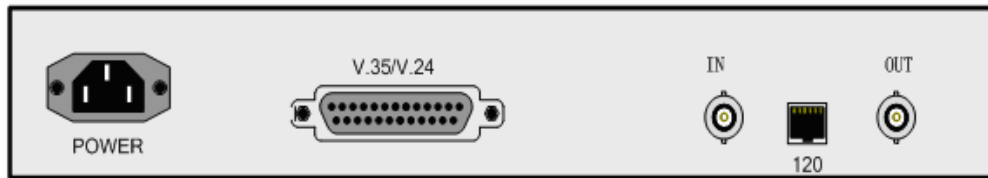
DA-2000 E1/V. 35 转换设备后面板
